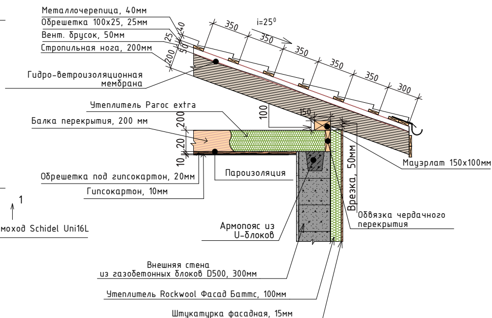
Схема устройства деревянной скатной крыши газобетонного дома с деревянным чердачным перекрытием
