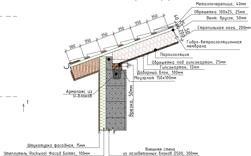
Схема устройства деревянной скатной крыши газобетонного дома без чердачного перекрытия
